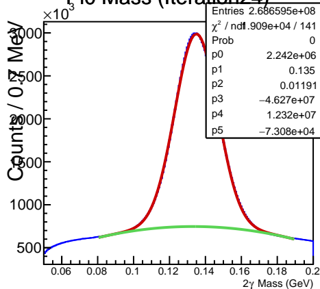
Pi0 Mass (Iteration24)
