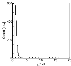
• \chi^2 distribution
