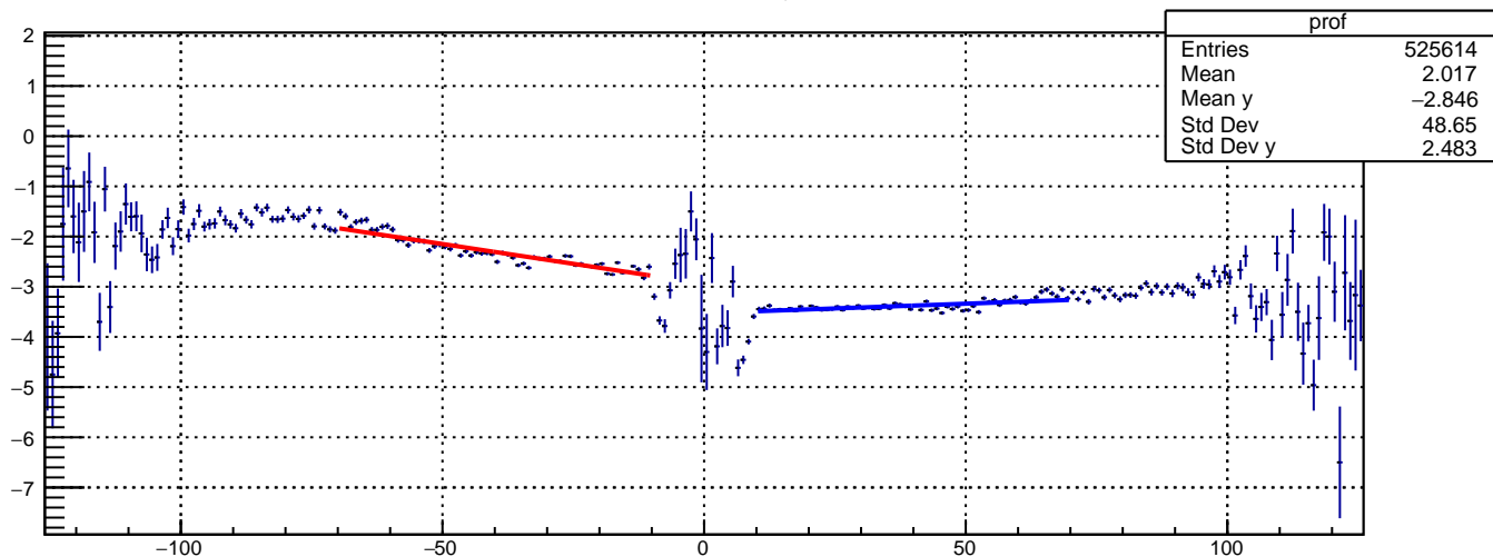
HorizontalPlaneQP21
