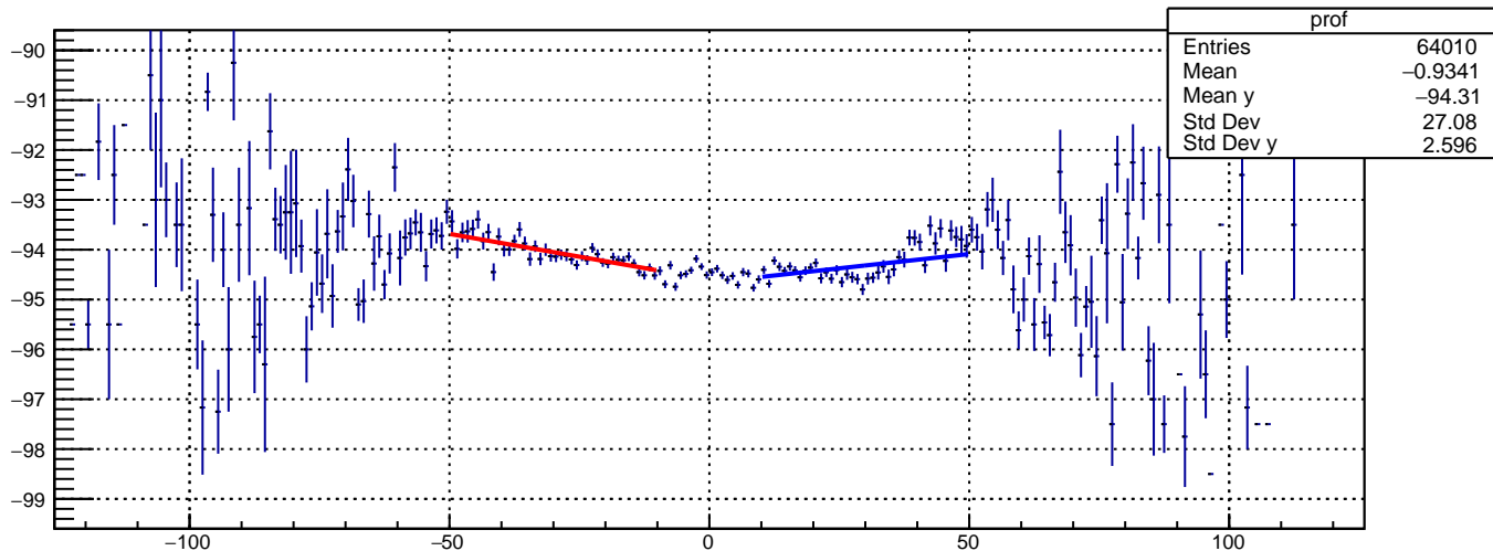
HorizontalPlaneQP5
