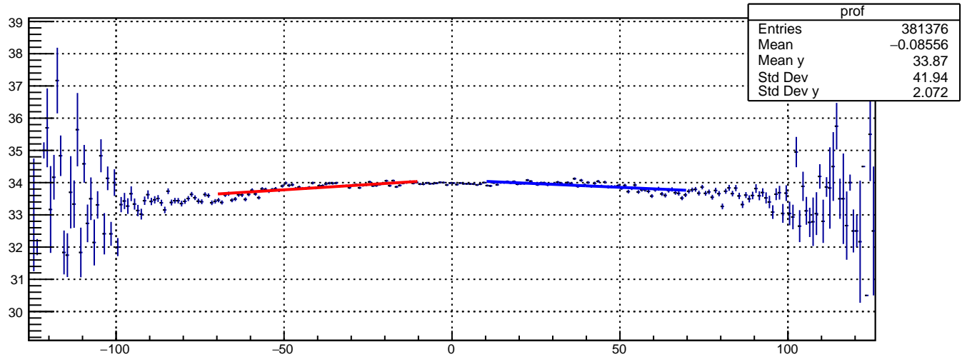
VerticalPlaneQM28
