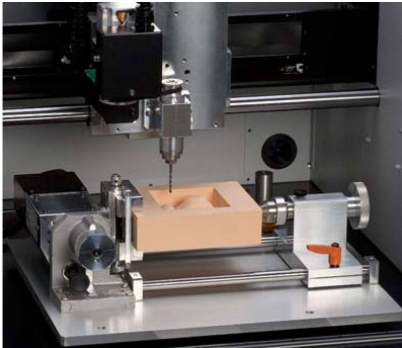
Sistema de eje rotativo.
