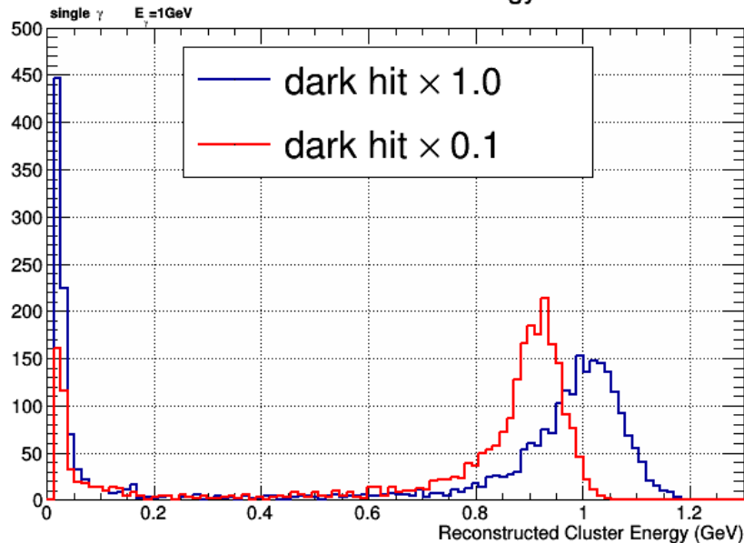
DBCALCluster Energy
