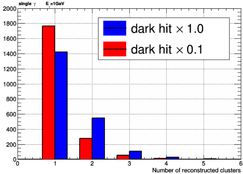
Num. DBCALClusters
