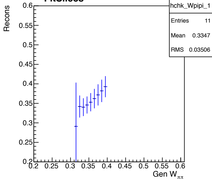
FitSlices
