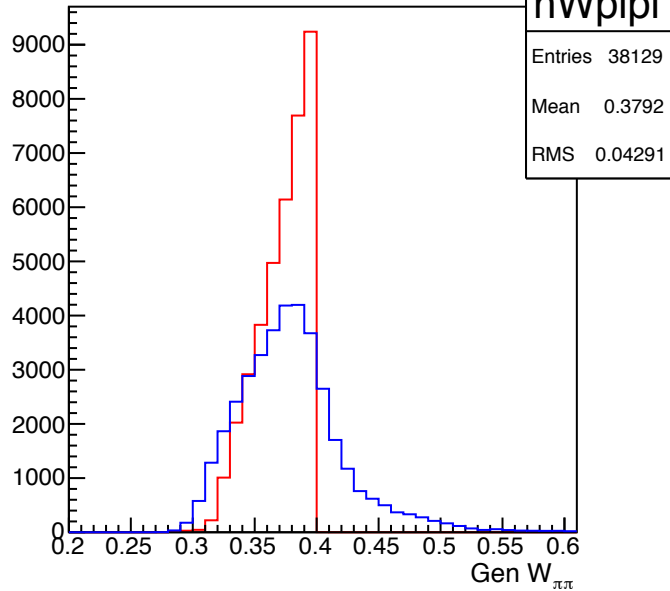
hWpipi
