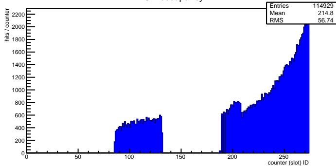
TAGH occupancy
